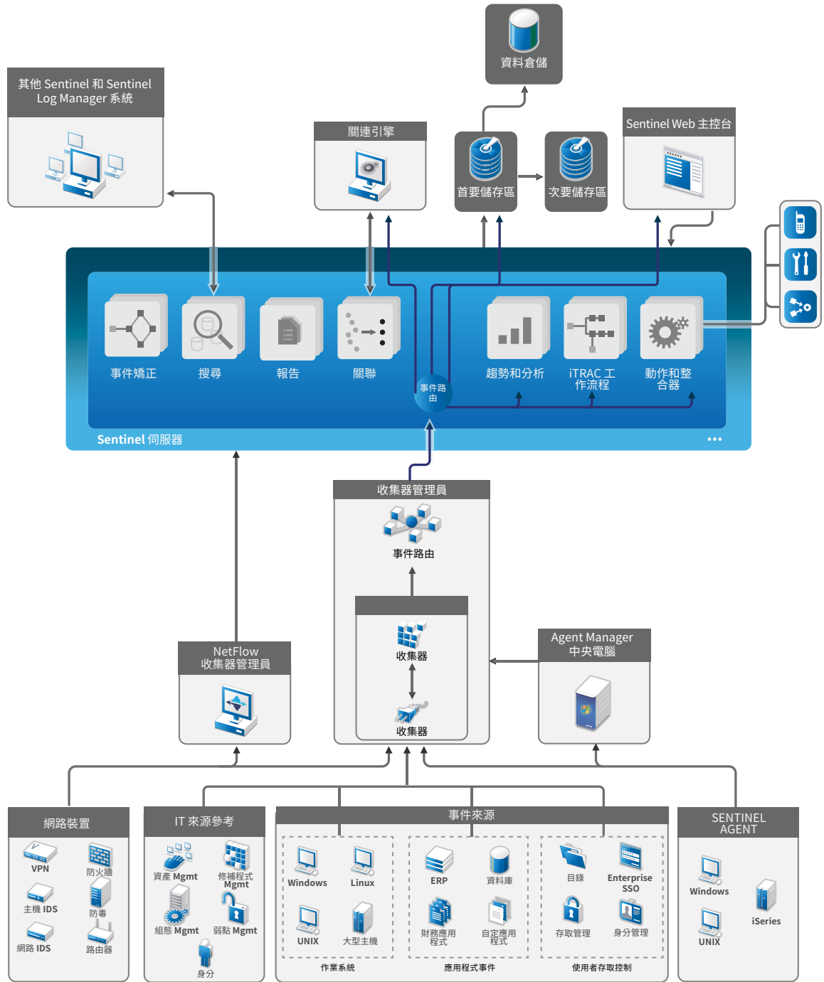
圖 2-1 Sentinel 架構
