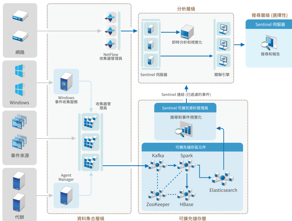
圖 6-6 可擴充儲存的三層部署
