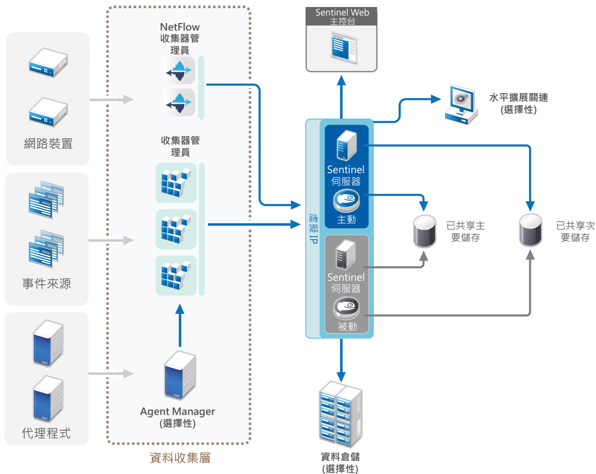
圖 6-4 高可用性單層分散式佈署
