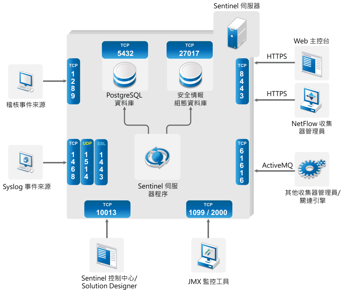
圖 8-1 Sentinel 中使用的連接埠
