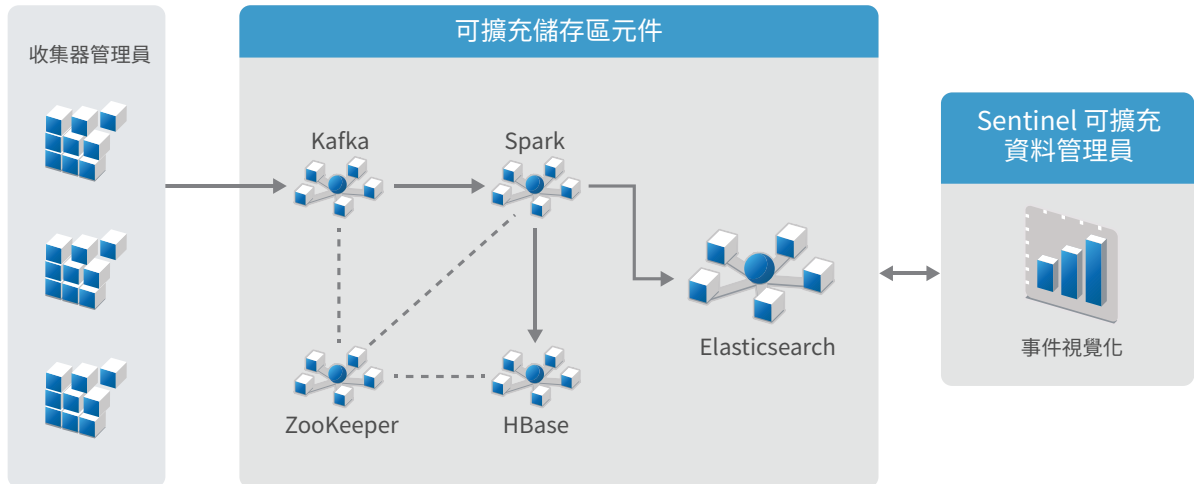
圖 6-1 可擴充儲存架構
