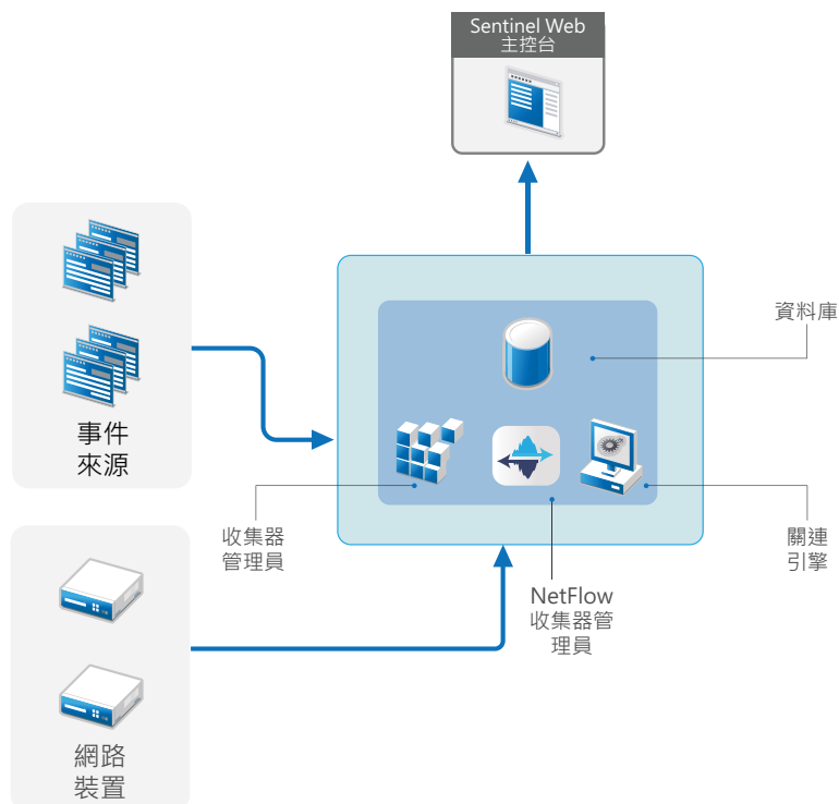
圖 6-2 整合式佈署
