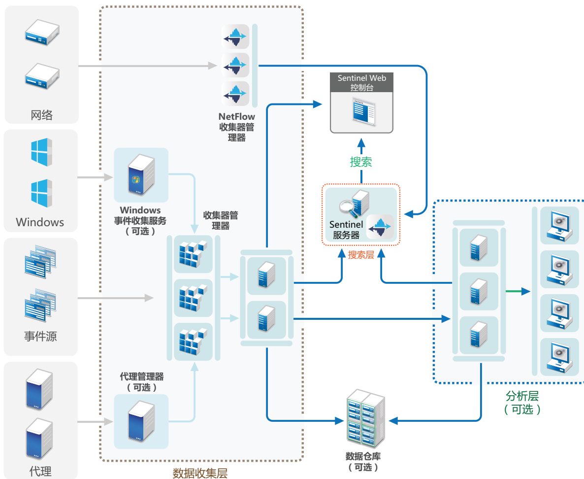
图 6-4 两层和三层分布式部署
