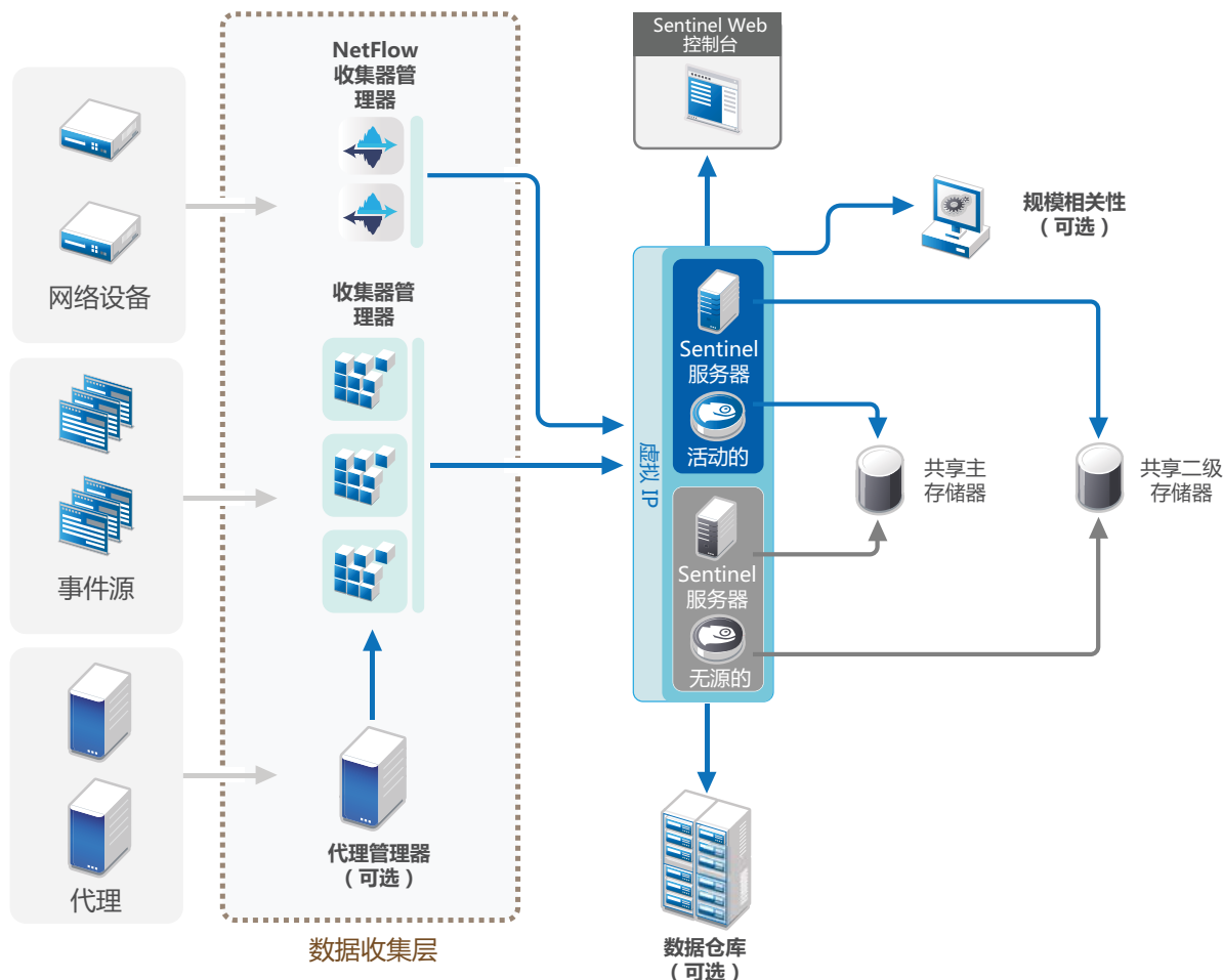
图 6-3 具有高可用性的一层分布式部署
