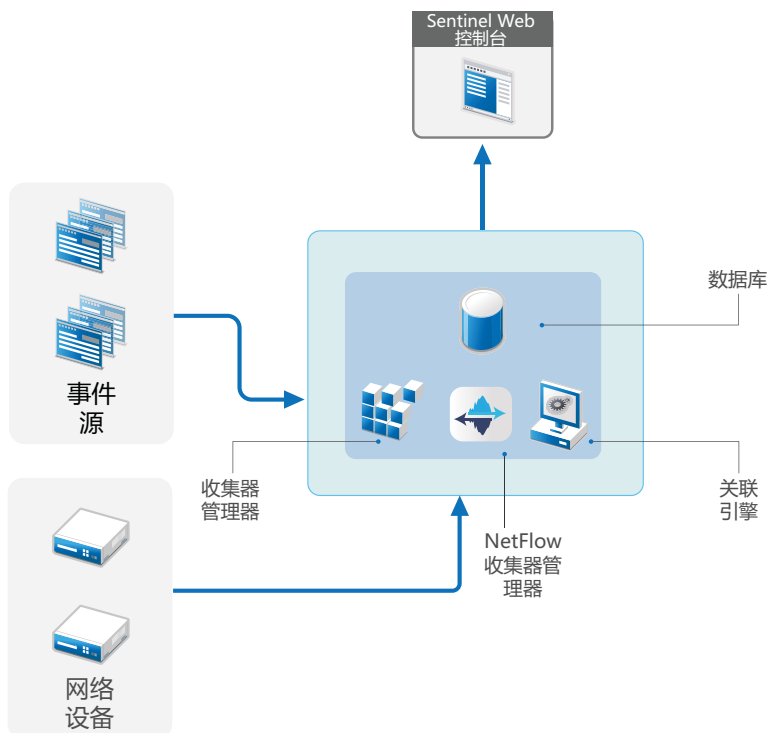
图 6-1 一体机部署
