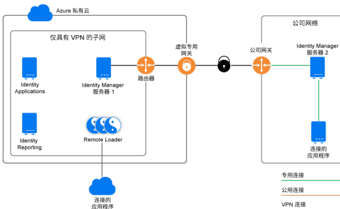
图21-1 使用多服务器驱动程序集连接的混合方案
