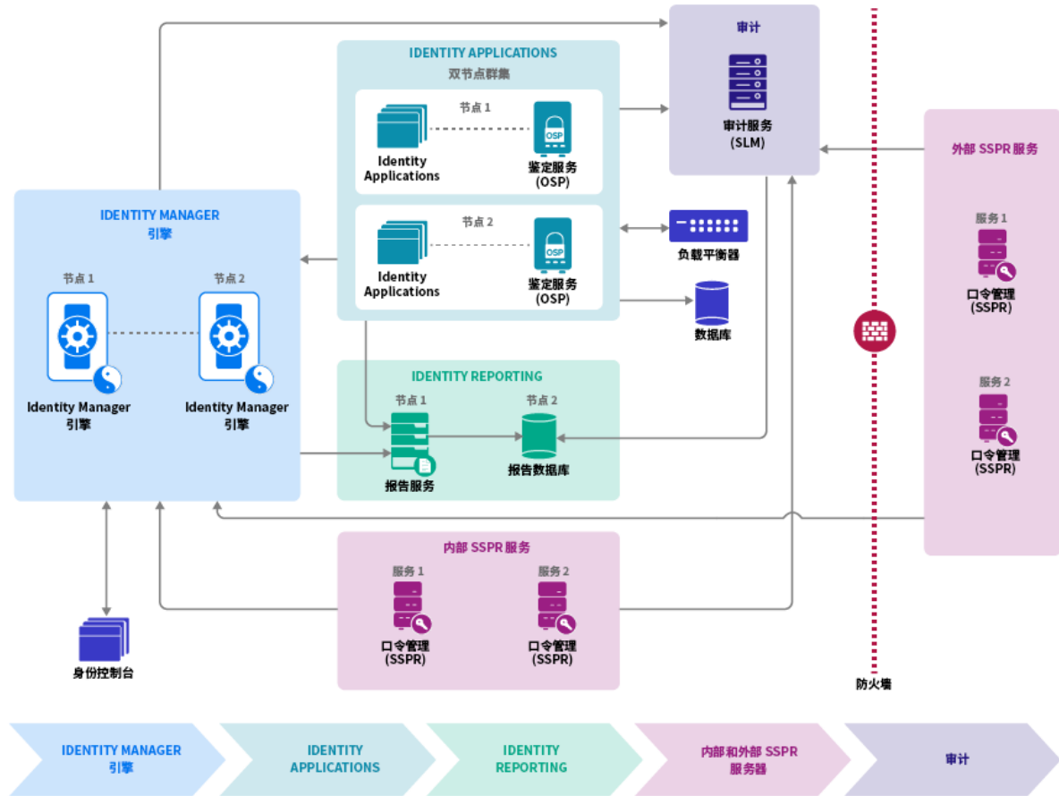
图1-4 高级版部署示例
