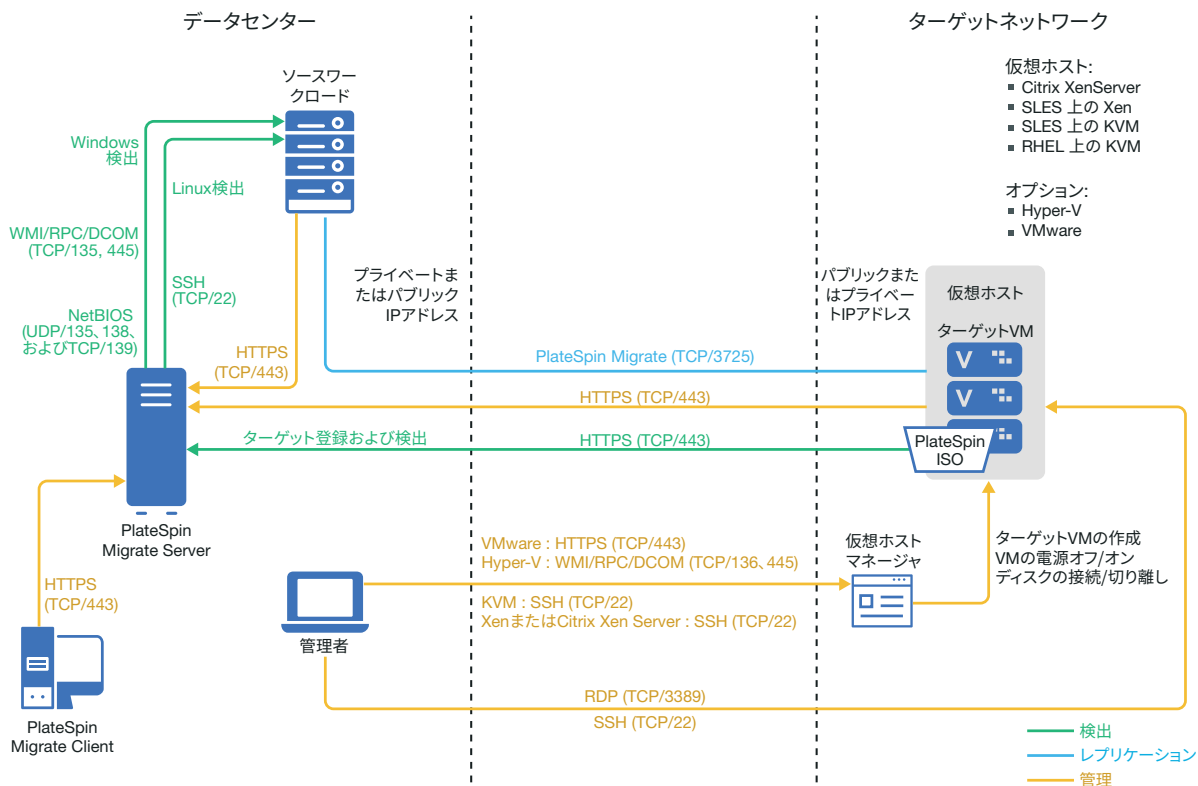
図 12-2 Hyper-V 上の VM への半自動マイグレーション
