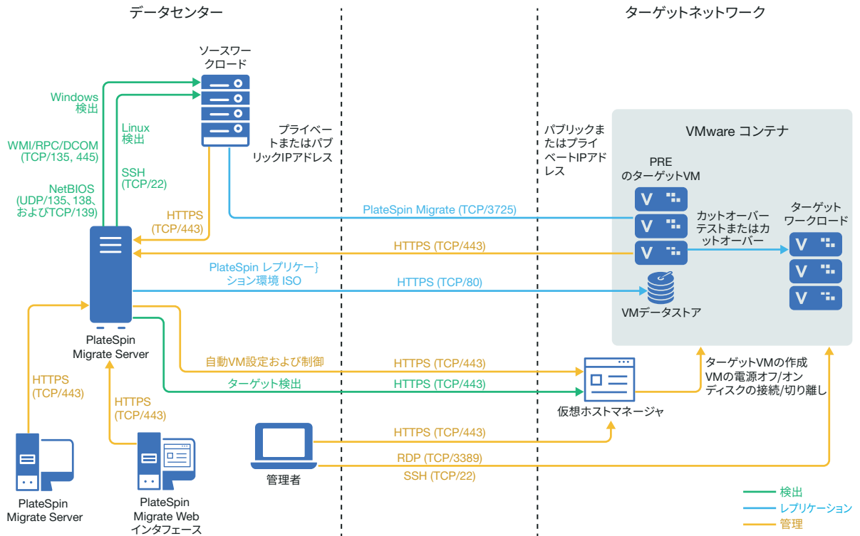
図 11-1 VMware への自動マイグレーション
