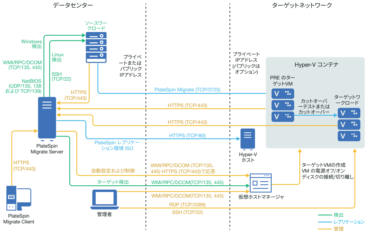
図 12-1 Hyper-V への自動マイグレーション
