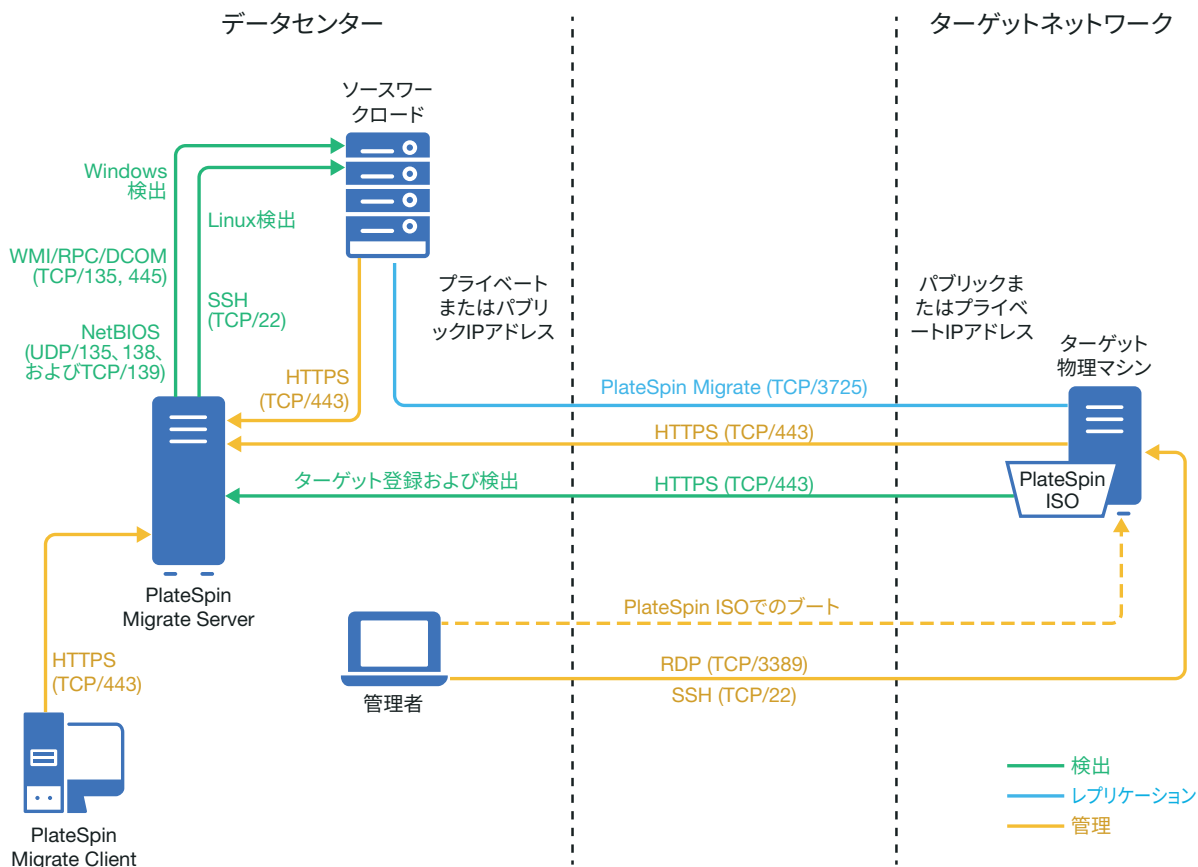
図 16-1 物理マシンへの半自動マイグレーション
