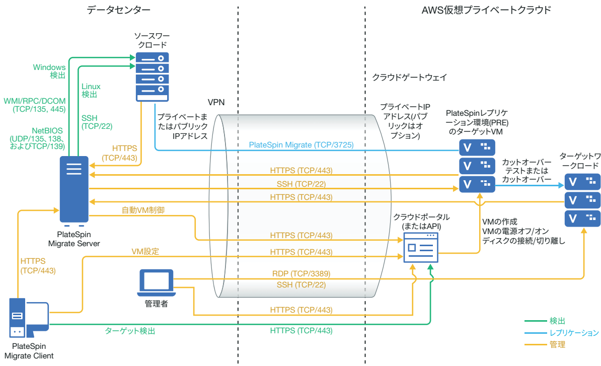
図 8-1 AWS への半自動マイグレーション用のオンプレミス Migrate サーバ
