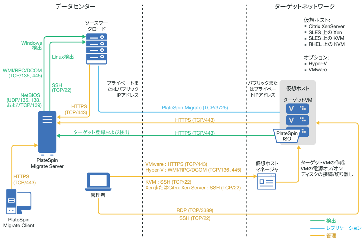
図 15-1 KVM 上の VM への半自動マイグレーション
