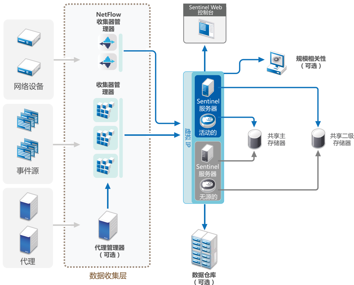
图 6-3 具有高可用性的一层分布式部署
