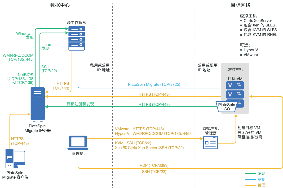
图 16-1 以半自动化方式迁移到 KVM 上的 VM
