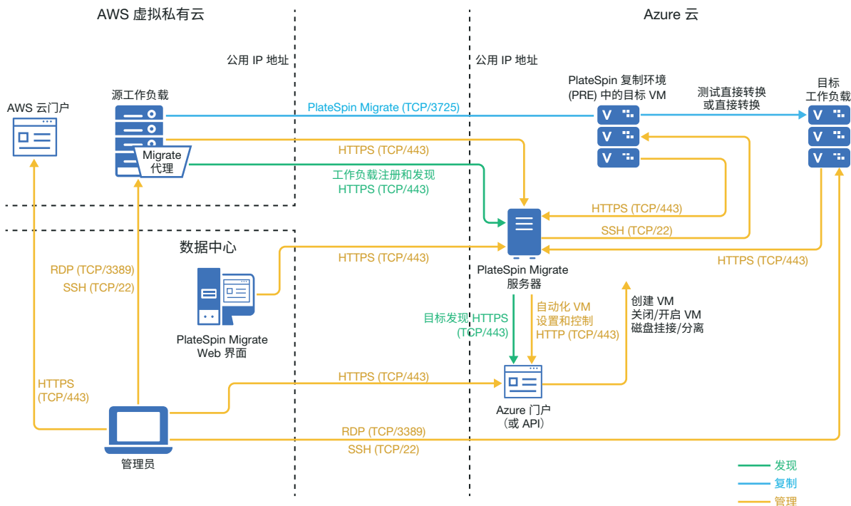
图 10-1 用于从 AWS 自动迁移到 Azure 的基于云的 Migrate 服务器
