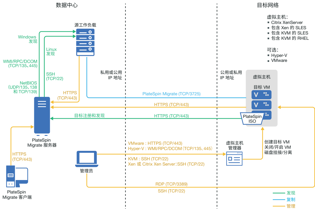
图 12-2 以半自动化方式迁移到 VMware 上的 VM
