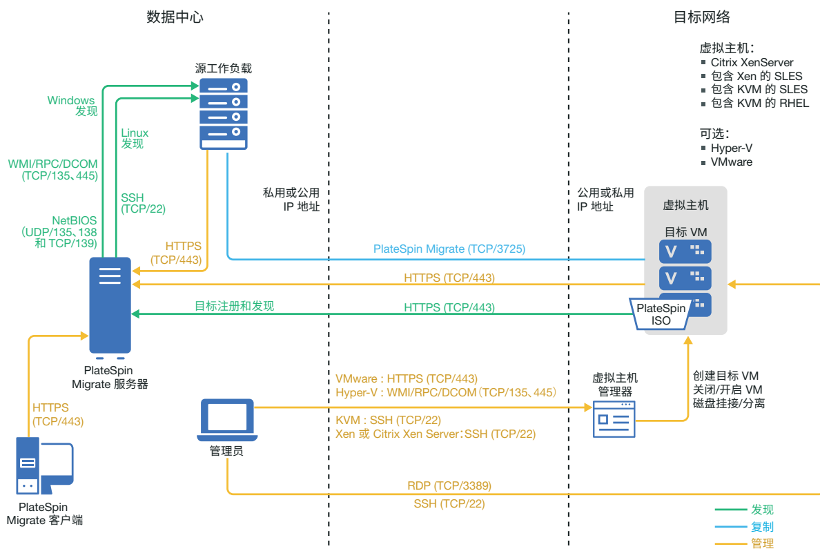
图 13-2 以半自动化方式迁移到 Hyper-V 上的 VM
