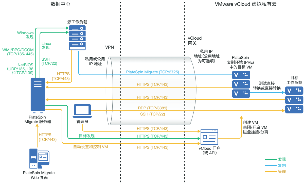
图 11-1 用于自动迁移到 vCloud 的本地 Migrate 服务器
