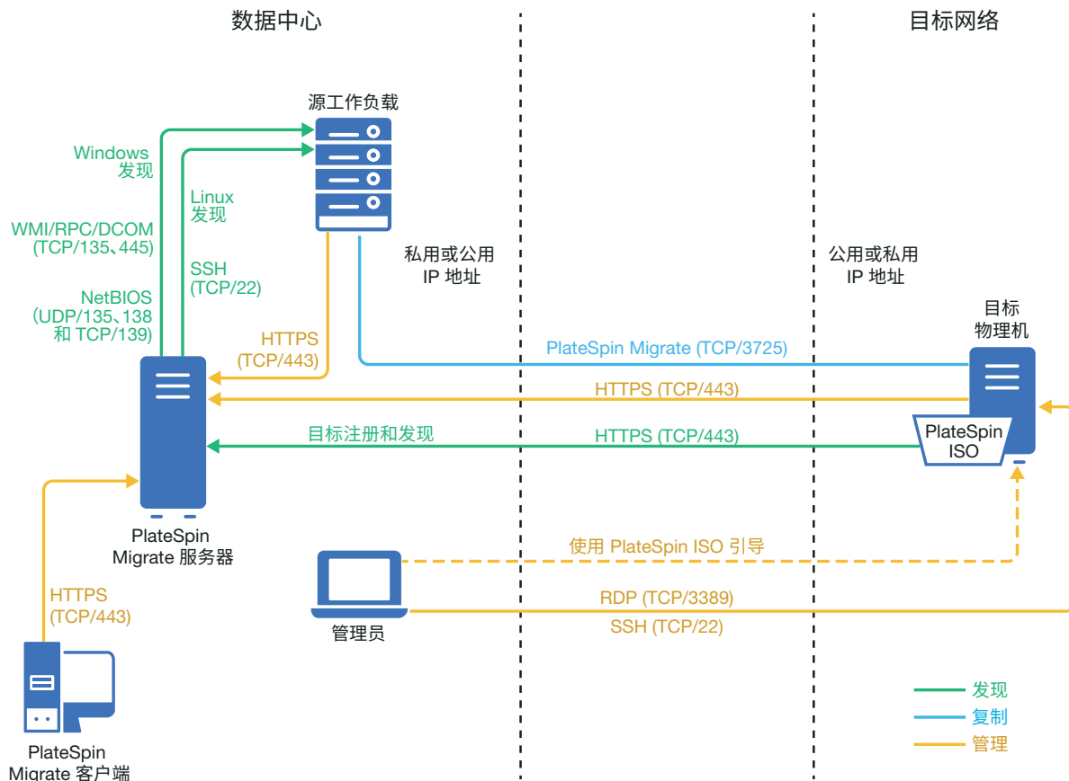
图 17-1 以半自动化方式迁移到物理机
