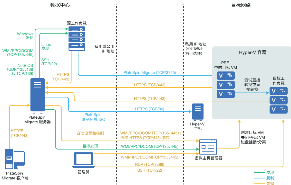
图 13-1 自动迁移到 Hyper-V
