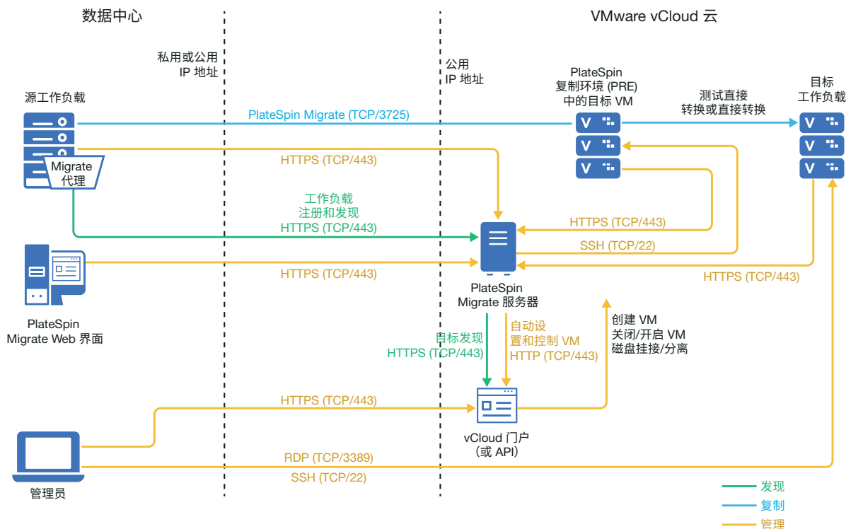
图 11-2 用于自动迁移到 vCloud 的基于云的 Migrate 服务器
