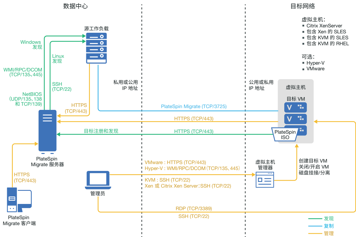
图 14-1 以半自动化方式迁移到 Citrix XenServer 上的 VM
