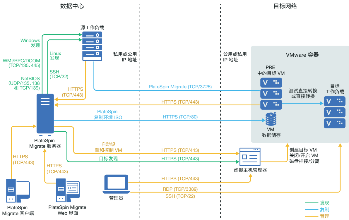
图 12-1 自动迁移到 VMware
