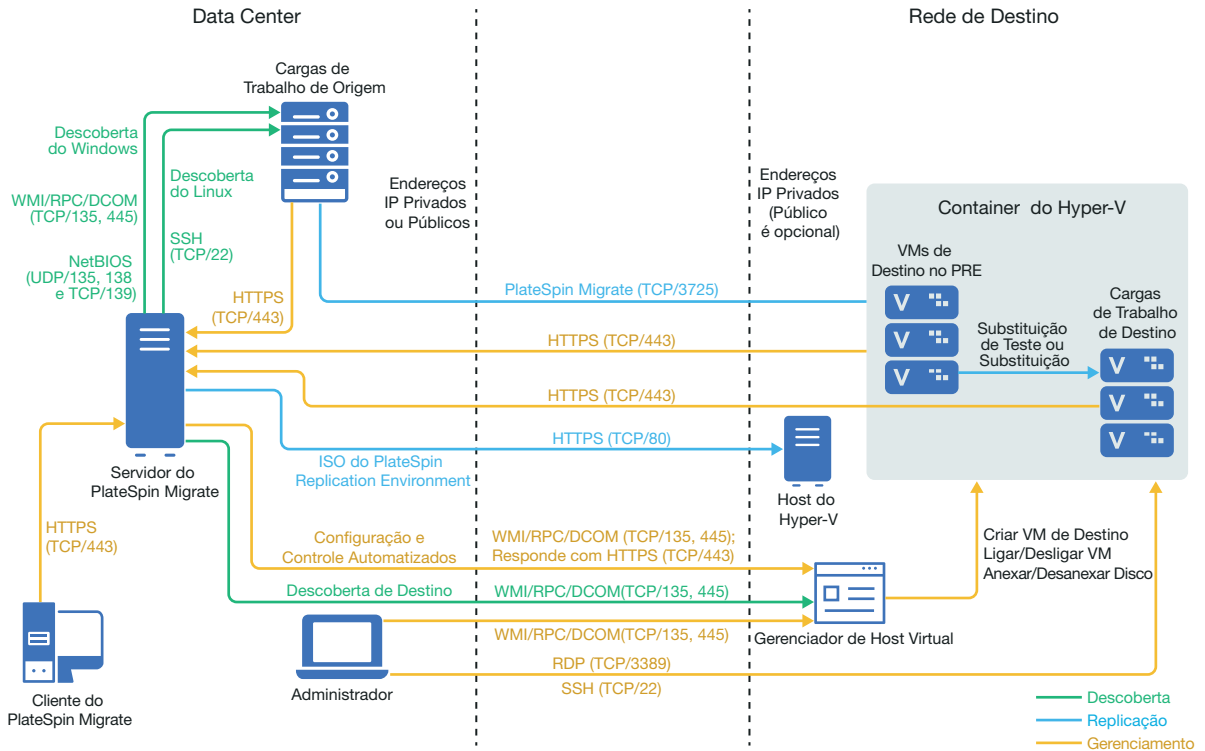
Figura 12-1 Migração Automatizada para Hyper-V
