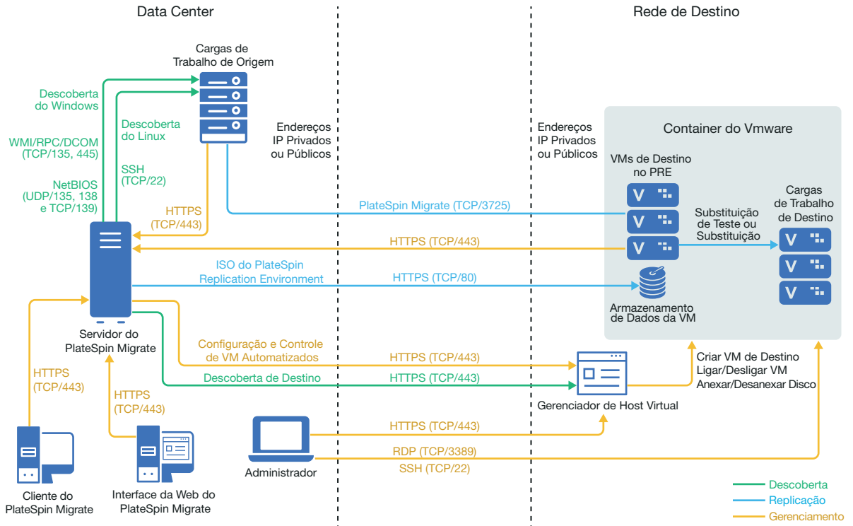
Figura 11-1 Migração Automatizada para VMware
