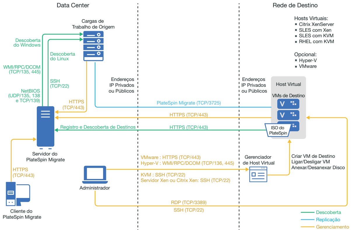
Figura 14-1 Migração Semiautomatizada para VMs no Xen
