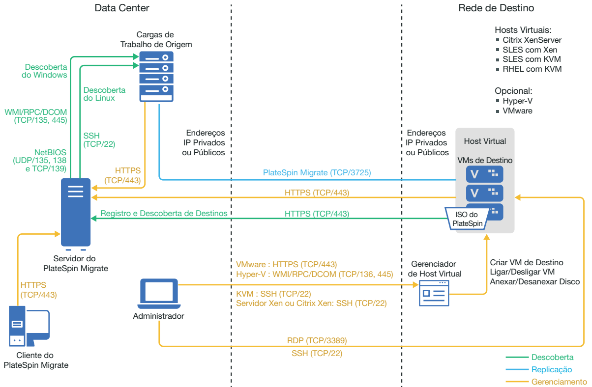
Figura 13-1 Migração Semiautomatizada para VMs no Citrix XenServer
