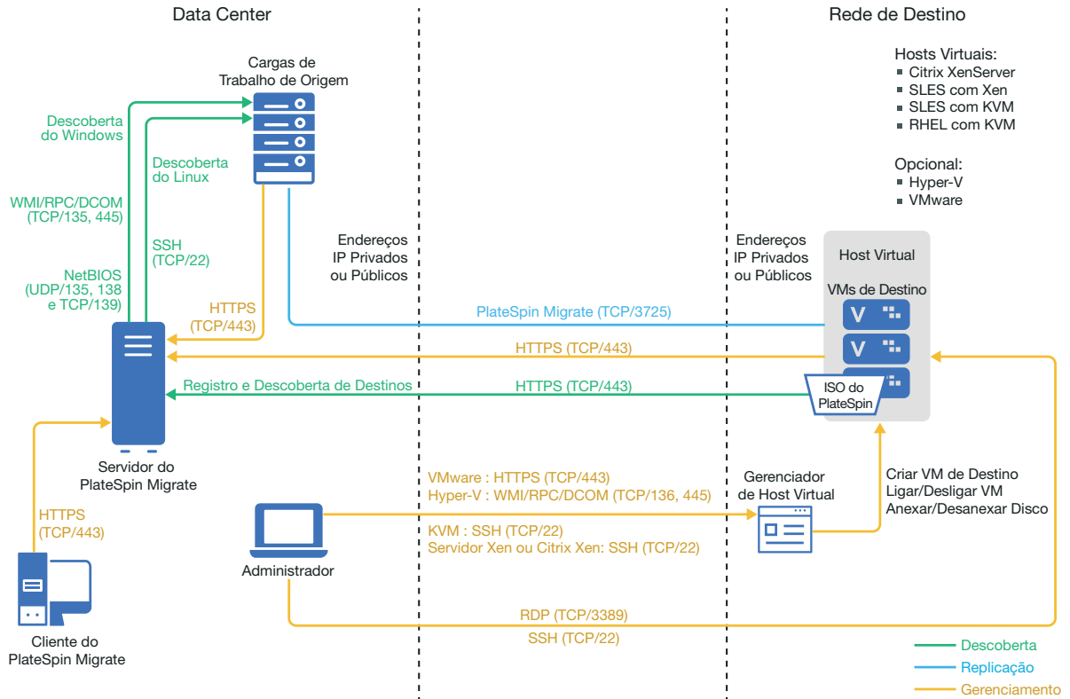
Figura 11-2 Migração Semiautomatizada para VMs no VMware
