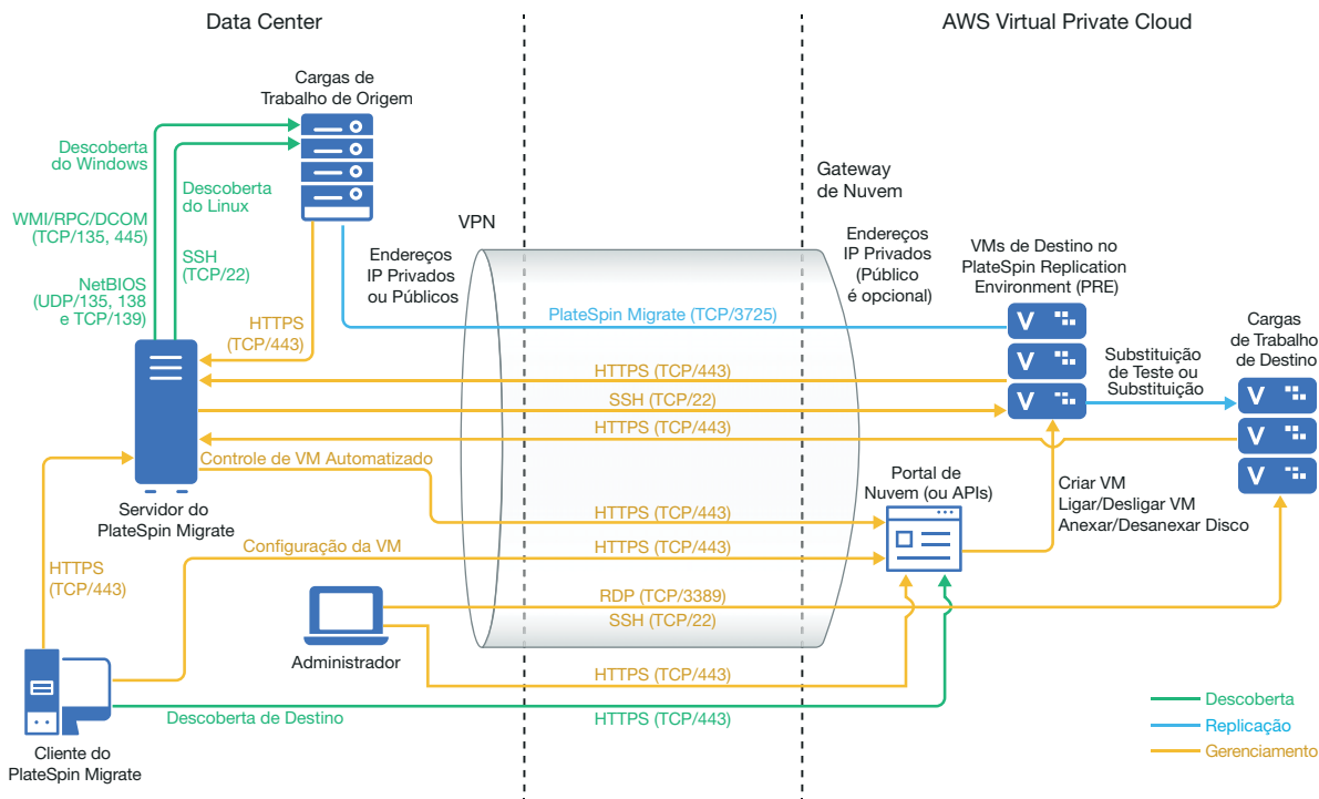
Figura 8-1 Servidor do Migrate no Local para Migração Semiautomatizada para AWS
