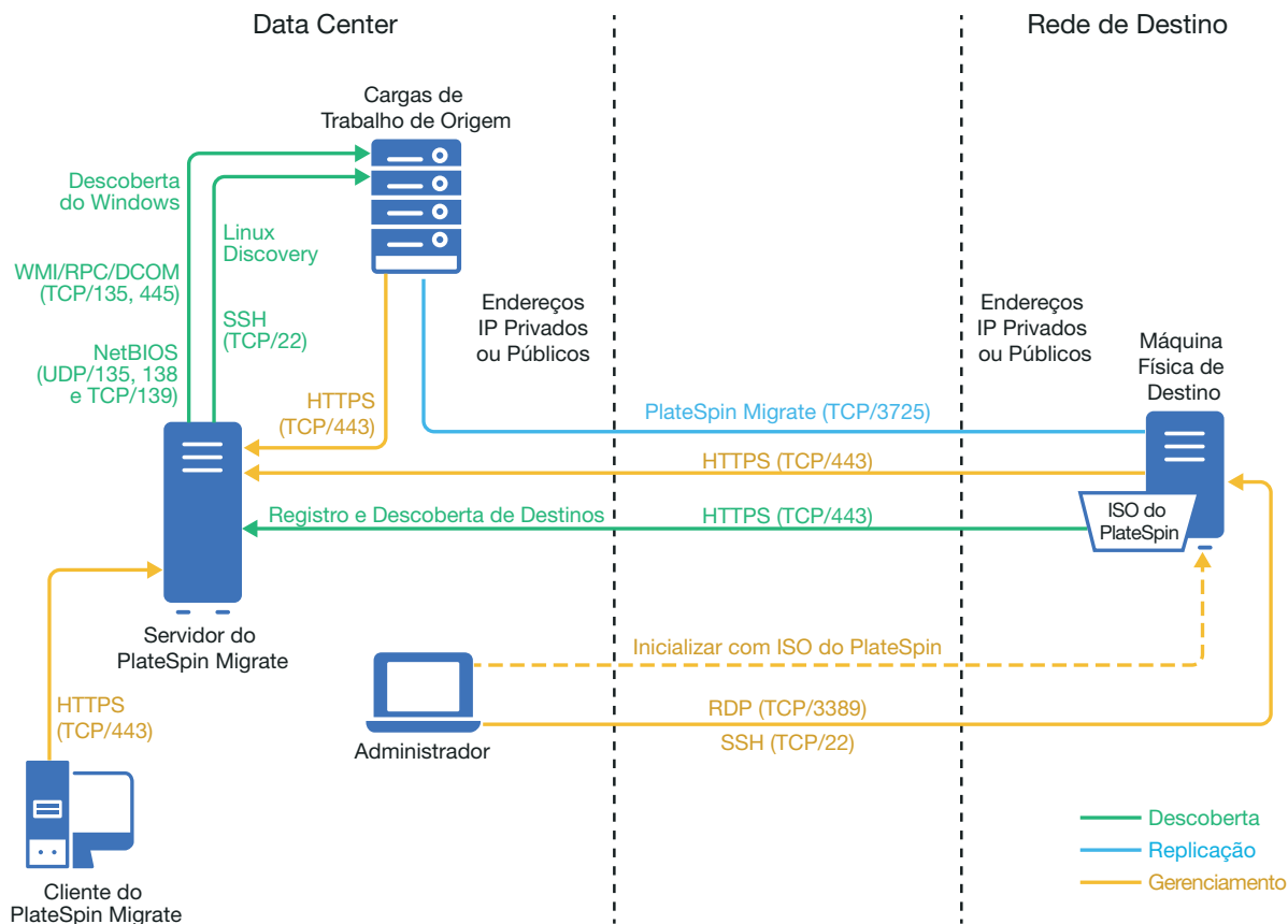
Figura 16-1 Migração Semiautomatizada para Máquinas Físicas
