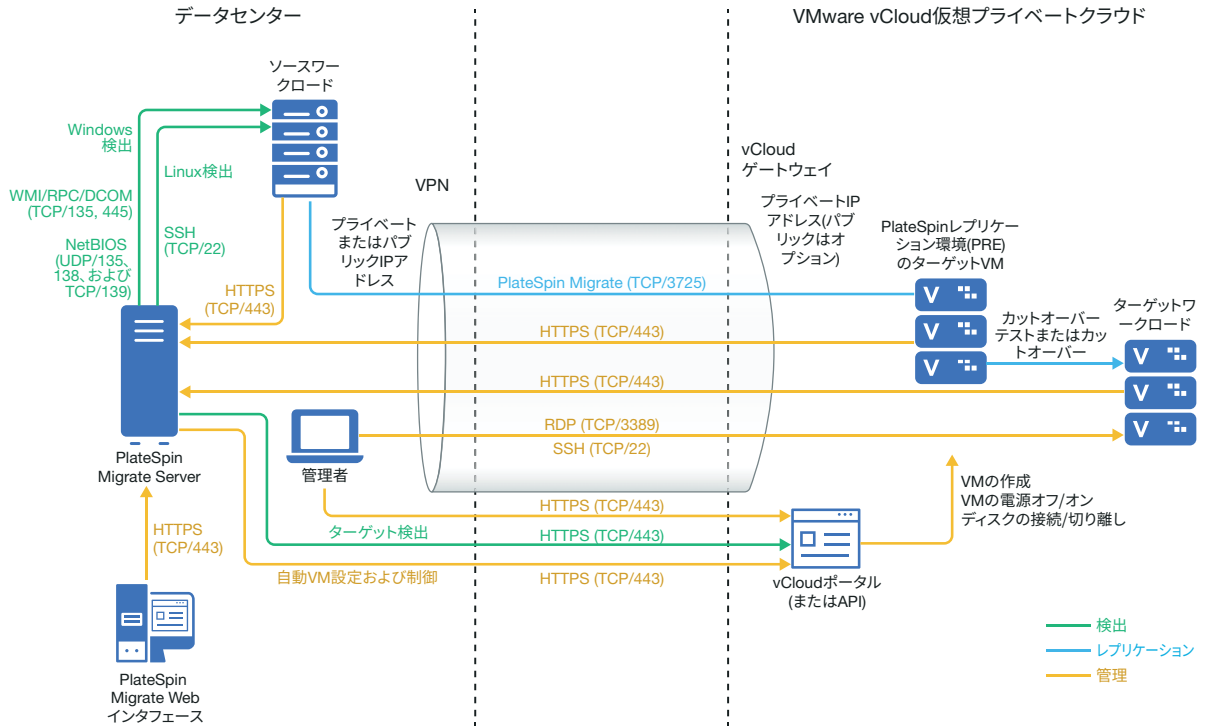
図 11-1 vCloud への自動マイグレーション用のオンプレミス Migrate サーバ
