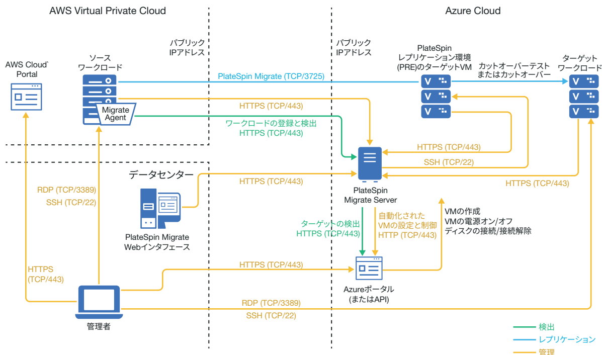
図 10-1 AWS から Azure への自動マイグレーション用のクラウドベース Migrate サーバ
