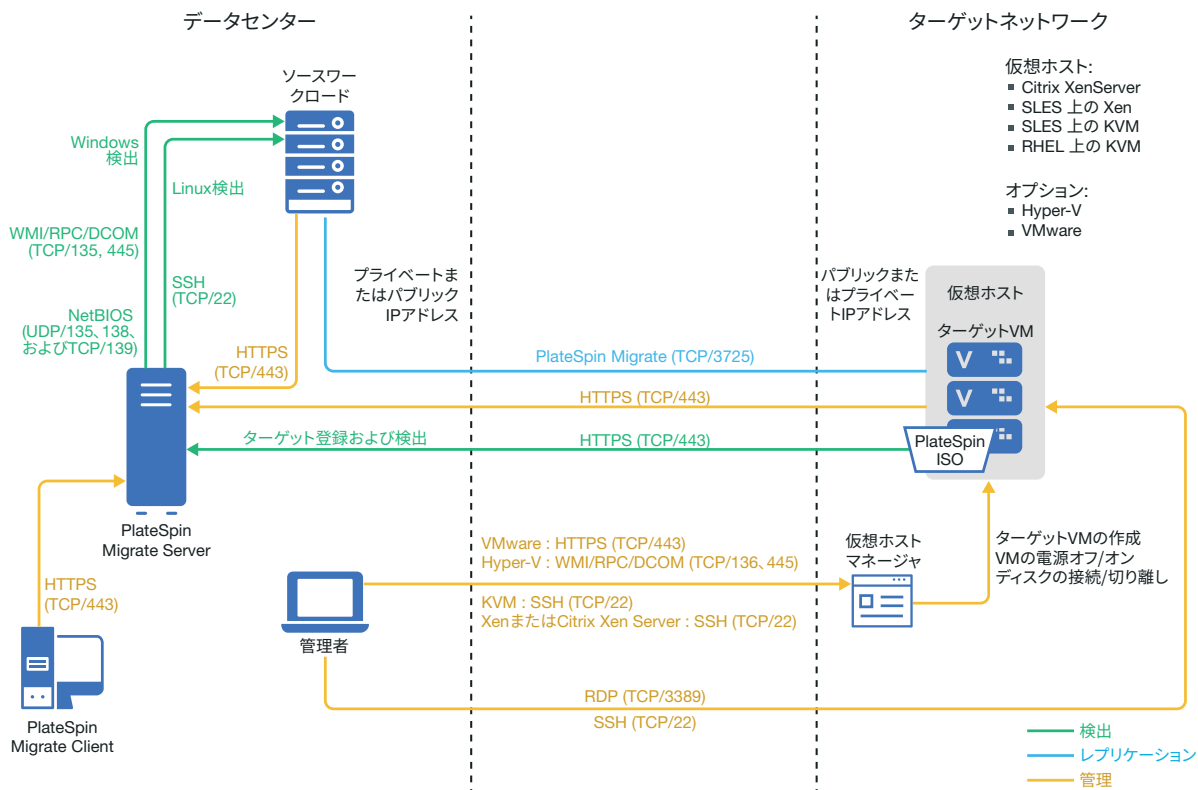
図 14-1 Citrix XenServer 上の VM への半自動マイグレーション
