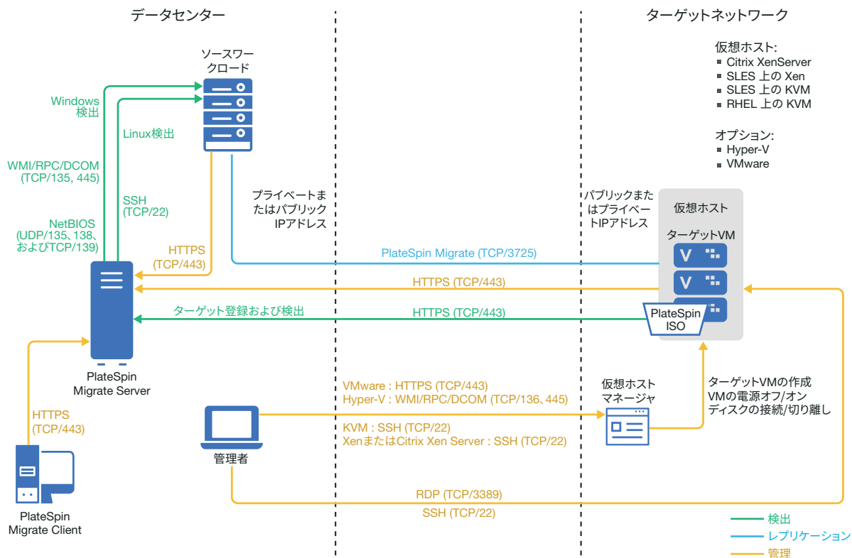
図 16-1 KVM 上の VM への半自動マイグレーション
