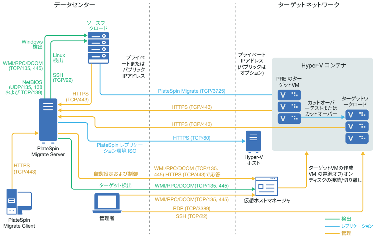
図 13-1 Hyper-V への自動マイグレーション
