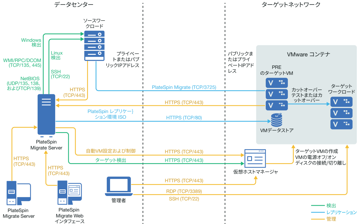
図 12-1 VMware への自動マイグレーション
