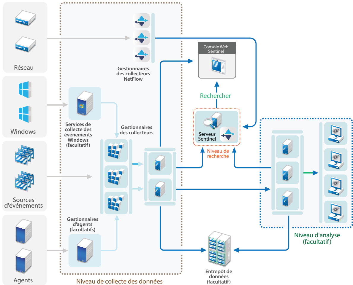
Figure 6-4 Déploiement distribué en deux ou trois niveaux
