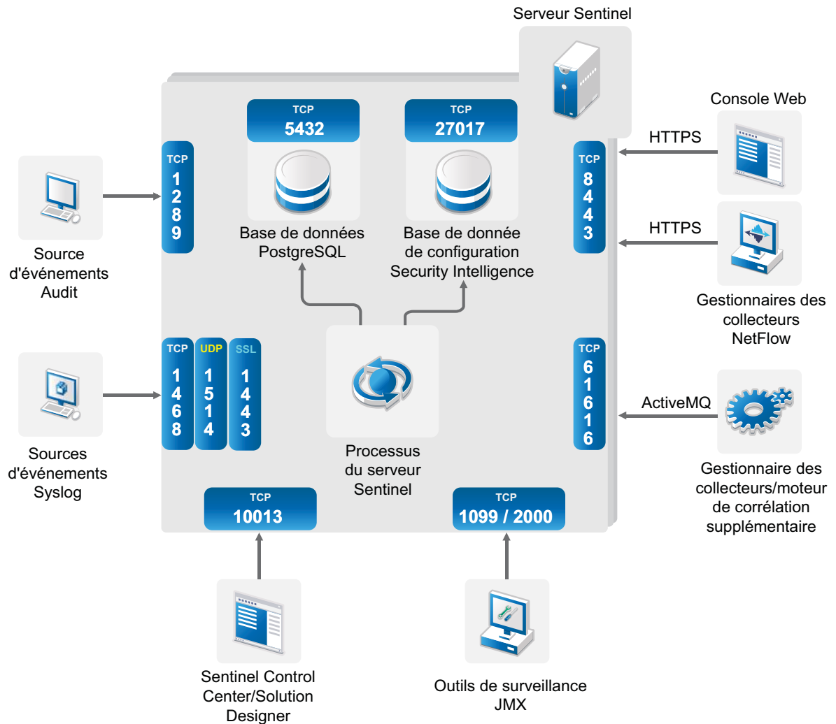
Figure 8-1 Ports utilisés dans Sentinel
