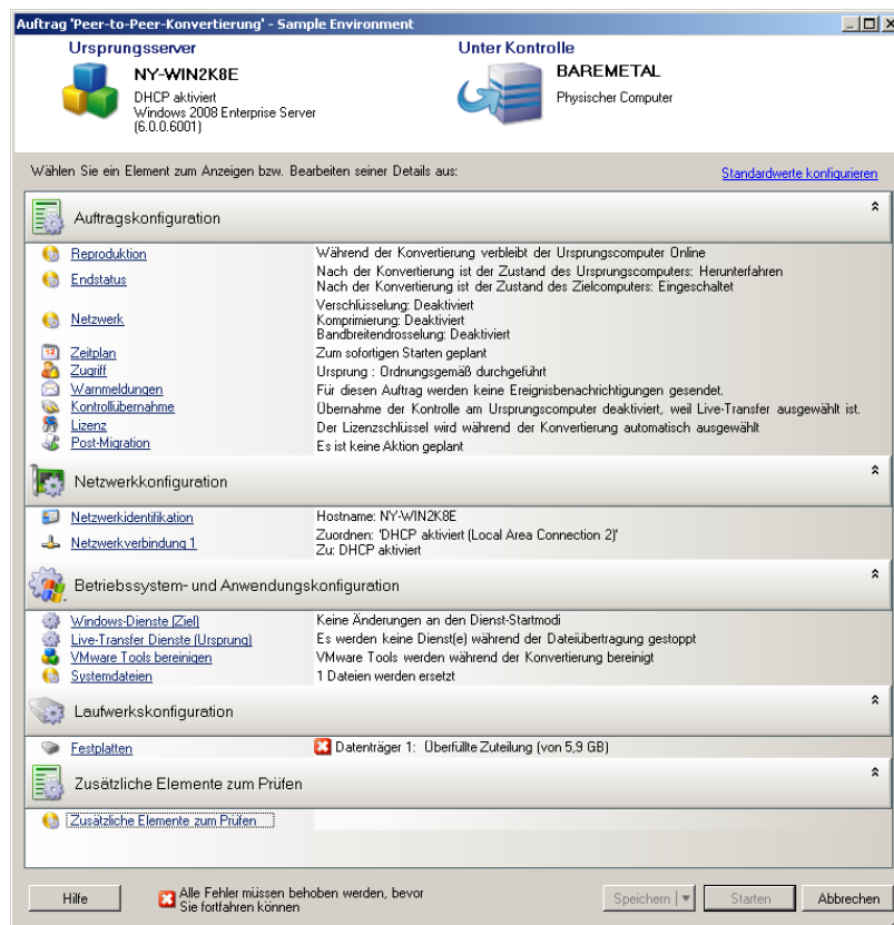
Abbildung 5-2 Fenster „Auftrag 'Peer-to-Peer-Konvertierung'“ (V2P im erweiterten Modus)
