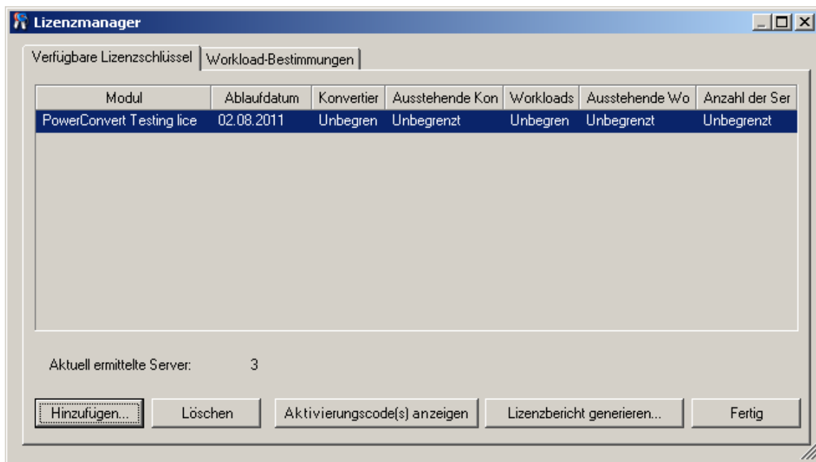
Abbildung 2-2 Verfügbare Lizenzschlüssel
